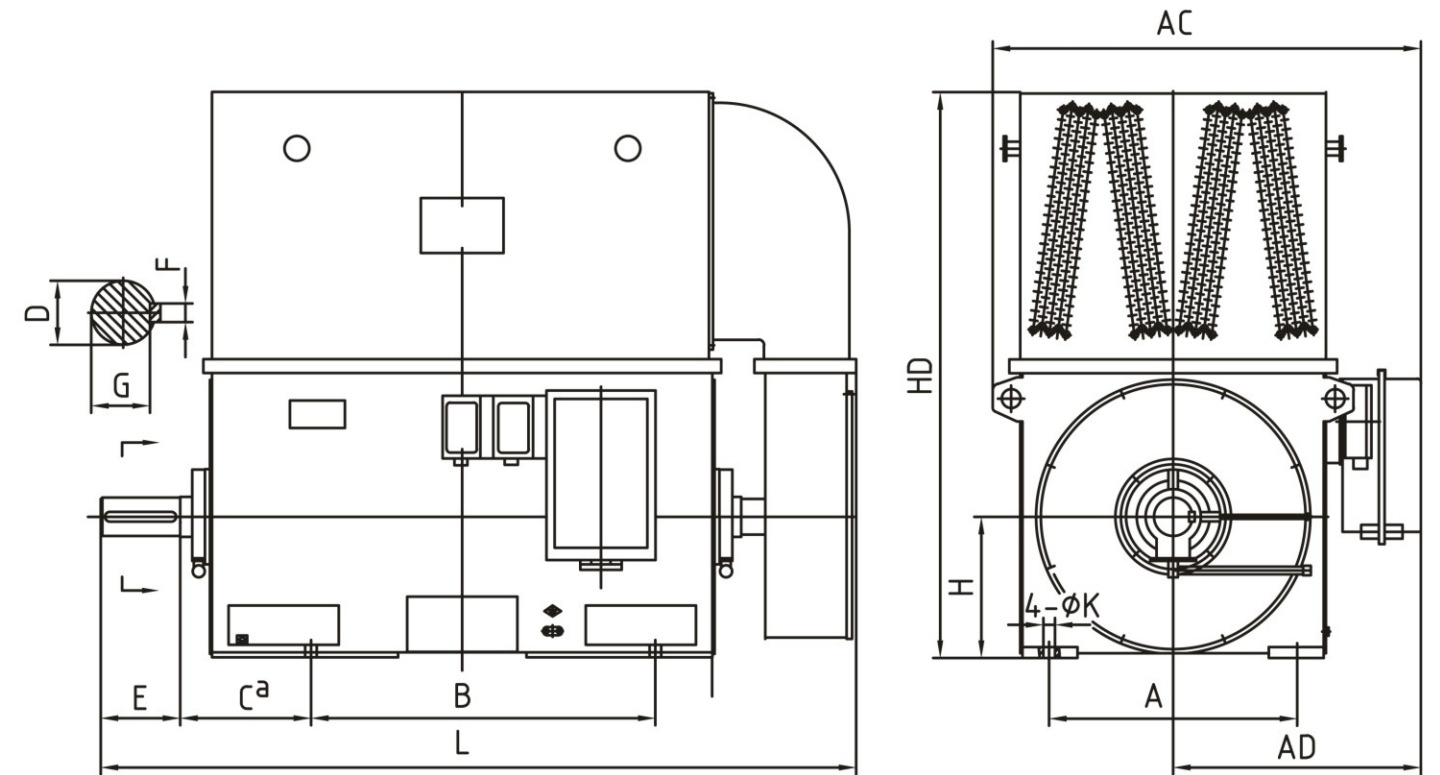
YXKK系列 (6kV) 中型高压三相异步电动机外形尺寸图
